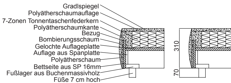
Querschnittsansicht Boxunterbau SC51:
