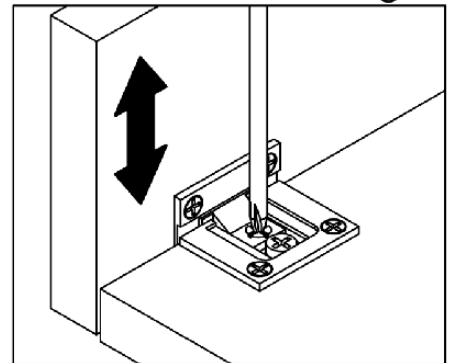
Höhenverstellung
