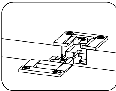
Seitenverstellung
