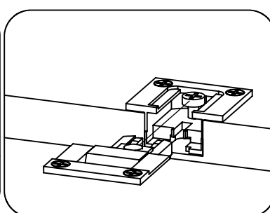
Seitenverstellung
