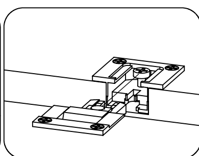
Seitenverstellung
