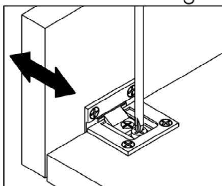
Tiefenverstellung
