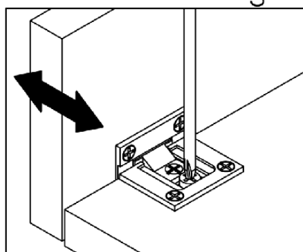
Tiefenverstellung
