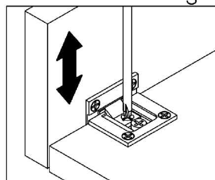
Höhenverstellung
