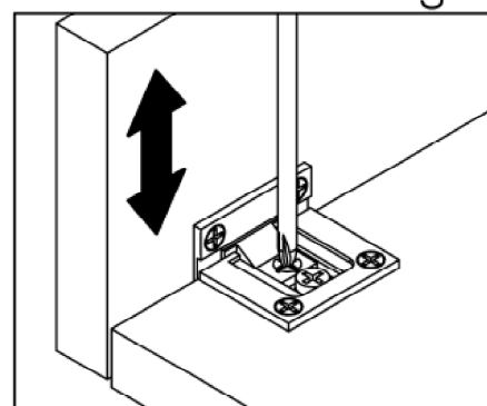
Höhenverstellung
